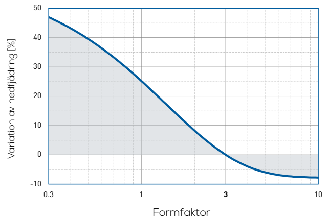
Nedfjädring
