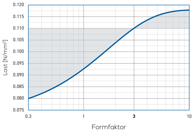
Statiskt belastningsområde
