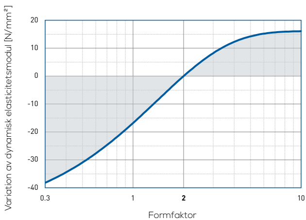
Dynamisk elasticitetsmodul vid 10 Hz
